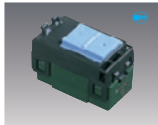
WT5001 希望小売価格190円 税抜 埋込スイッチB(片切) AC15A 300V
